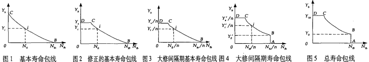
图1 基本寿命包线
