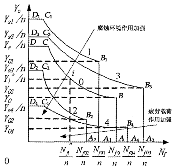
图6 非基准使用条件下结构大修间隔期包线
